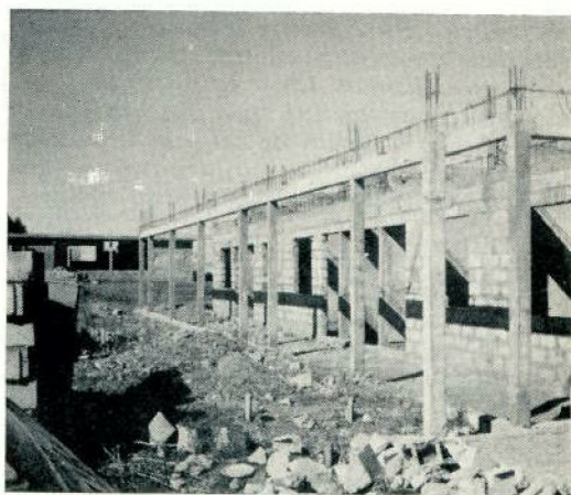
Estado de las obras del hospital de Thiés
